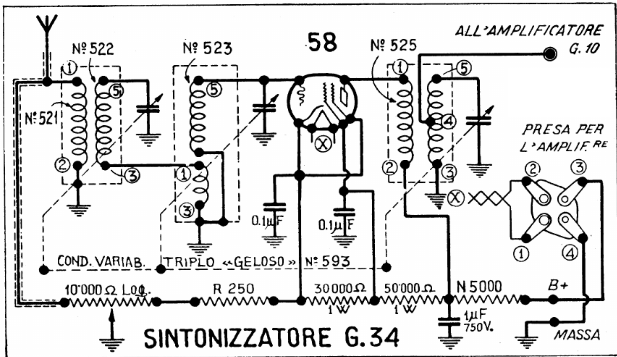
- Lo schema elettrico del sintonizzatore G 34.
